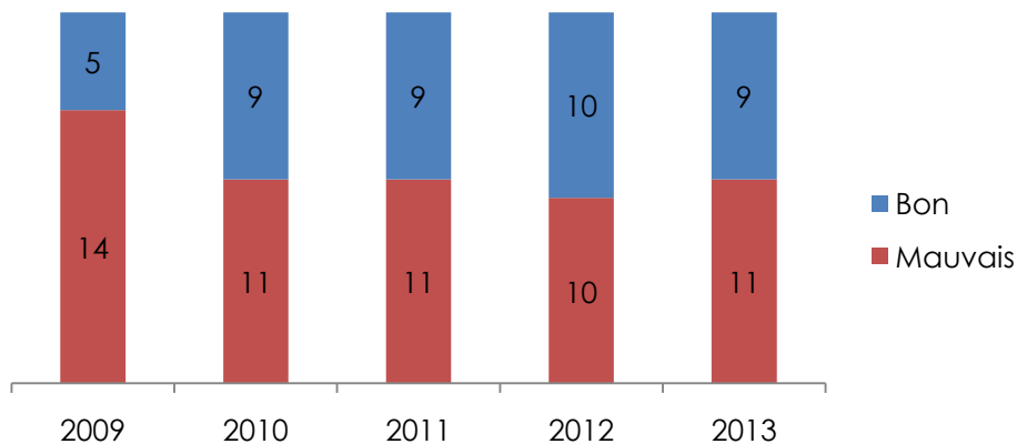
Evolution du nombre de stations déclassées par les pesticides de 2009 à 2013
