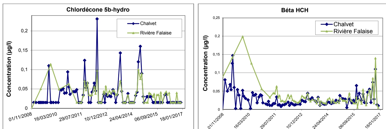
Illustration 30 : Fluctuations mensuelles mesurées sur Basse Pointe – Rivière Falaise pour la chlordécone 5 b-hydro et le bêta HCH (les valeurs inférieures à la limite de quantification sont représentées comme égales à LQ/2)
