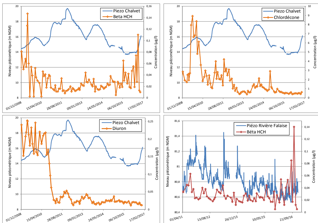
Illustration 32 : Fluctuations des concentrations en pesticides et du niveau piézométrique au droit des forages de Basse Pointe – Chalvet et Rivière Falaise
