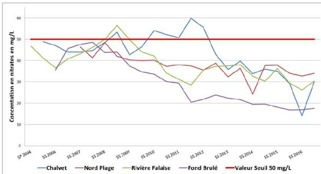
Illustration 14 : Evolution des nitrates pour les 4 stations les plus impactées du réseau
