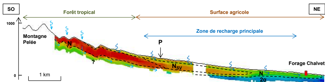
Illustration 22 : Coupe géophysique du bassin versant de Chalvet
