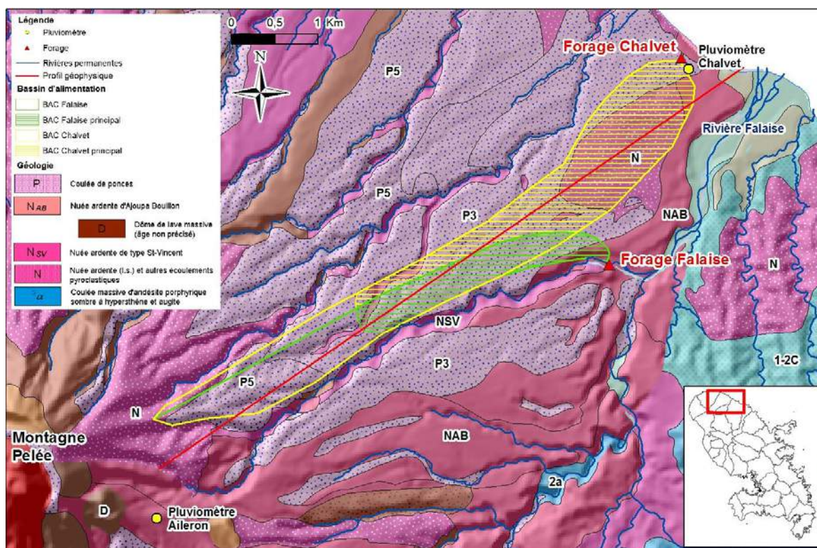
Illustration 21 : Délimitation approximative des bassins d'alimentation des forages Rivière Falaise et Chalvet (les zones hachurées correspondent aux principales zones de recharge) (Arnaud et al., 2013)
