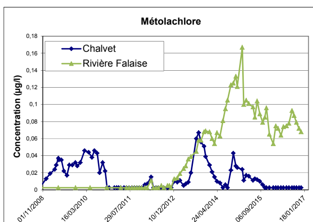
Illustration 31 : Comparaison des fluctuations mensuelles sur Chalvet et Rivière Falaise pour le métolachlore (les valeurs inférieures à la limite de quantification sont représentées comme égales à LQ/2)
