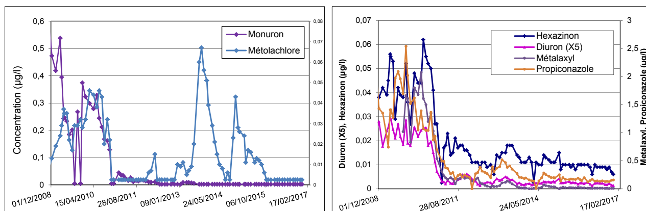
Illustration 27 : Fluctuations mensuelles mesurées sur Basse Pointe - Chalvet pour différents pesticides (les valeurs inférieures à la limite de quantification sont représentées comme égales à LQ/2)
