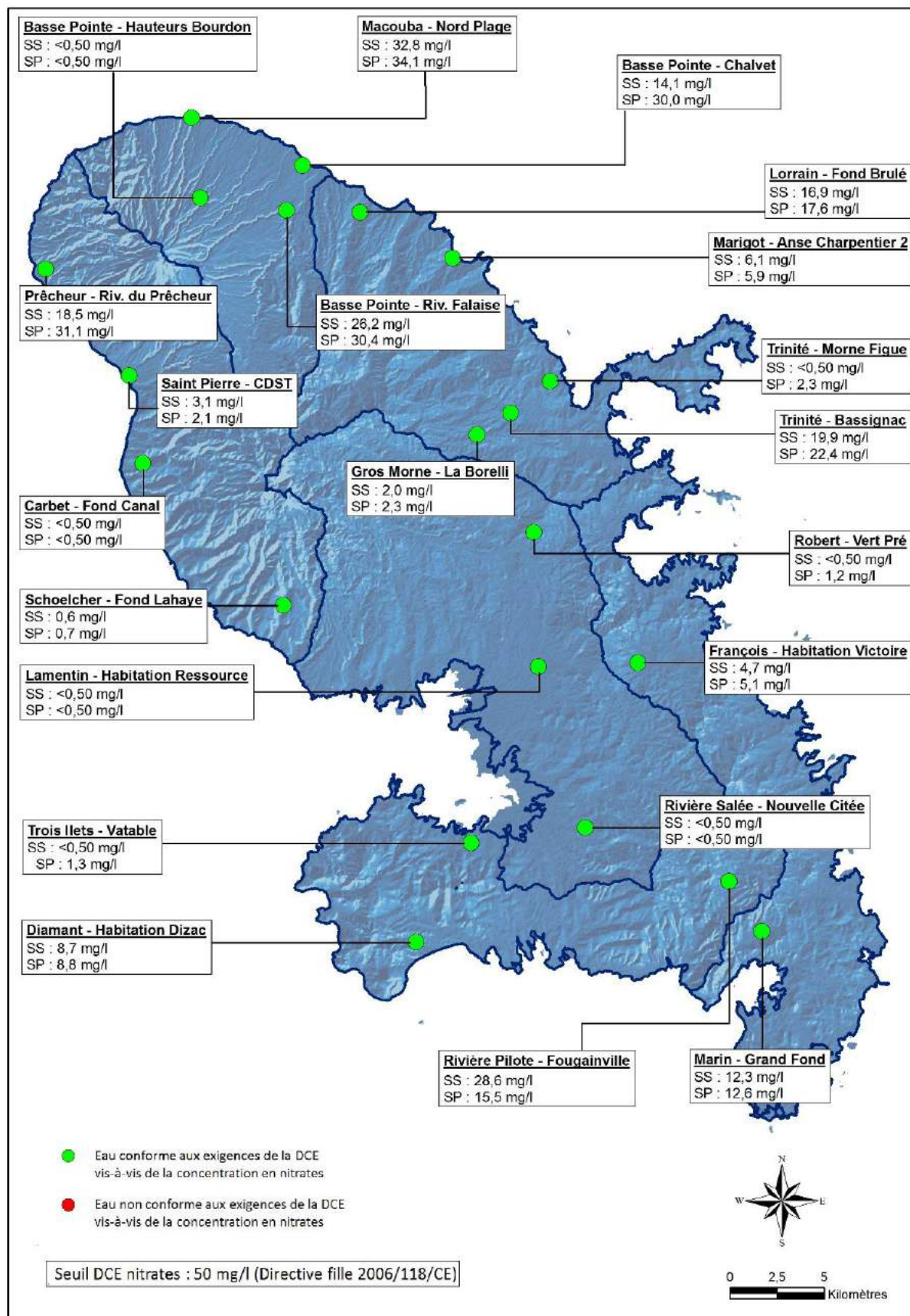
Illustration 10 : Concentrations en nitrates en saison sèche (SS) et saison des pluies (SP) 2016
