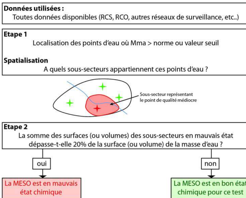
Illustration 7 : Test « qualité générale » permettant d'évaluer la proportion de la masse d'eau en bon état
