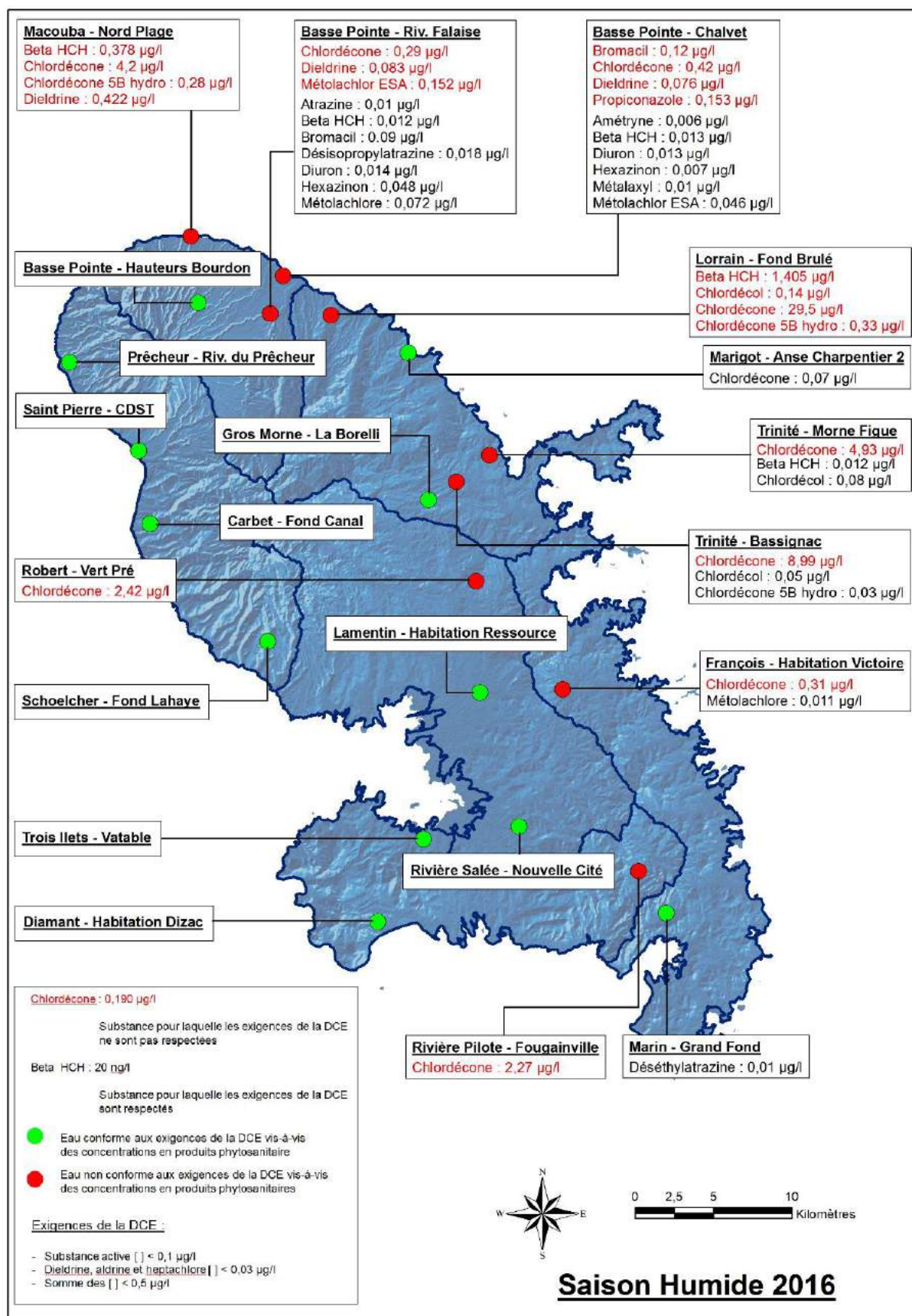
Illustration 12 : Produits phytosanitaires quantifiés en saison humide 2016
