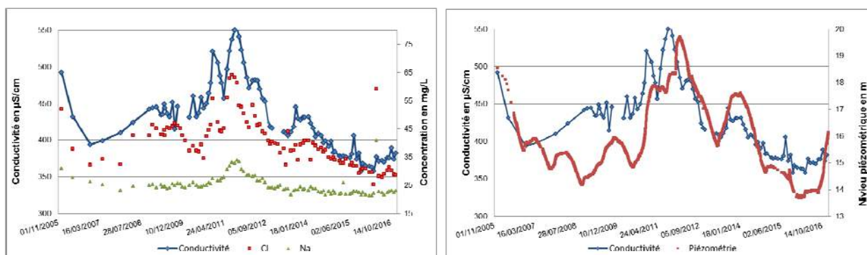
Illustration 24 : Évolution de la conductivité à Chalvet et des concentrations en sodium et chlorures (à gauche) et de la piézométrie (à droite)
