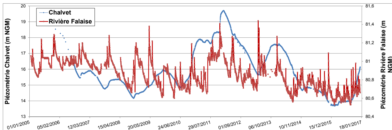
Illustration 20 : Chronique piézométrique des forages Chalvet (en bleu) et Rivière Falaise (en rouge) au pas de temps journalier (janvier 2005 – décembre 2016)
