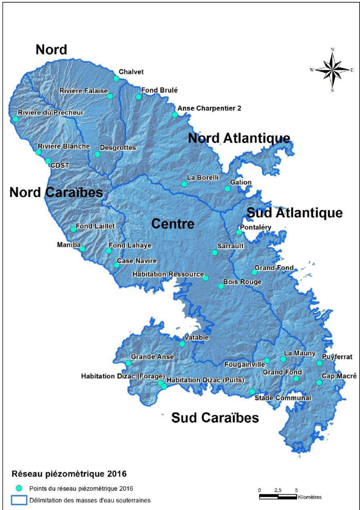
Illustration 2 : Carte de répartition des stations du réseau piézométrique de Martinique (état à fin décembre 2016)
