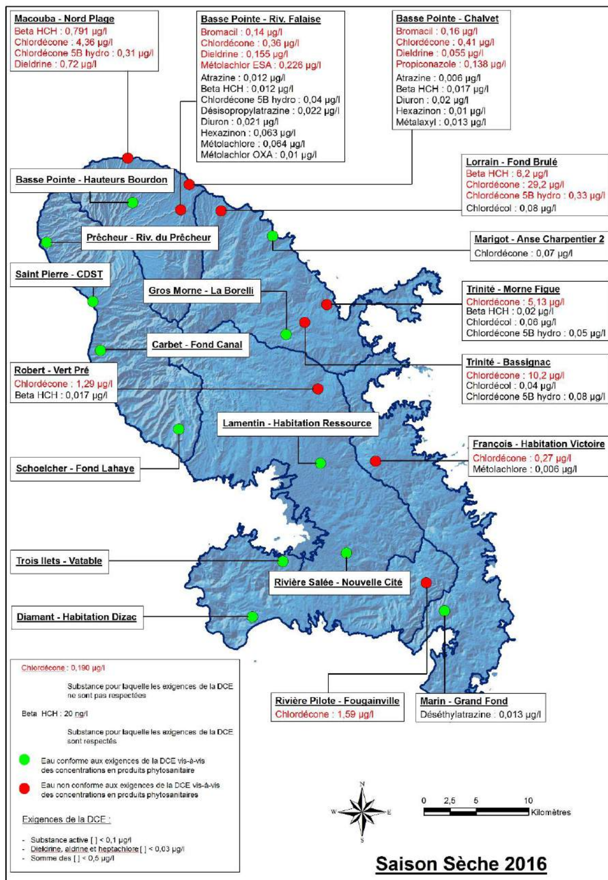
Illustration 11 : Produits phytosanitaires quantifiés en saison sèche 2016
