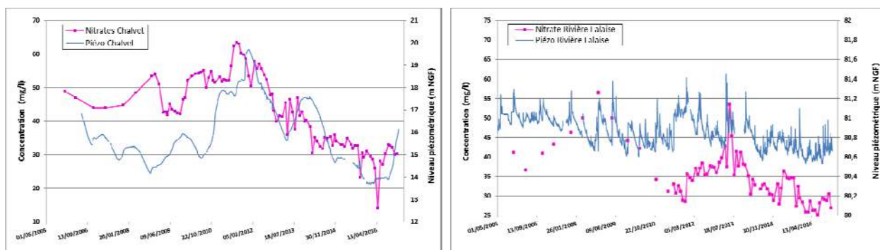
Illustration 25 : Fluctuations des concentrations en nitrates et du niveau piézométrique au droit des forages de Chalvet et de rivière Falaise
