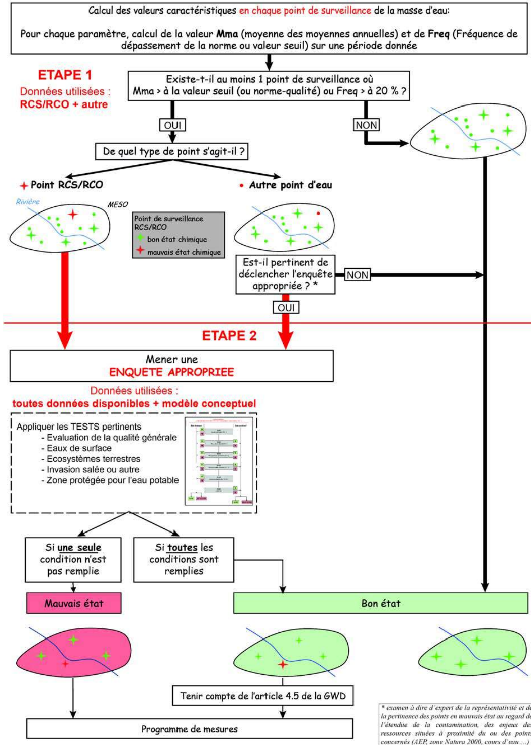
Illustration 6 : Procédure générale pour l'évaluation du bon état chimique d'une masse d'eau souterraine et application de l'enquête appropriée au titre de l'évaluation de l'état chimique (GWD : Groundwater Directive)
