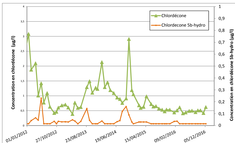
Illustration 28 : Fluctuations mensuelles mesurées sur Basse Pointe - Chalvet pour la chlordécone et la chlordécone 5b-hydro (les valeurs inférieures à la limite de quantification sont représentées comme égales à LQ/2)
