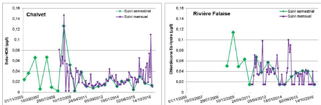
Illustration 26 : Évolution des concentrations en bêta HCH à Chalvet depuis décembre 2005 et des teneurs en chlordécone-5b-hydro à Rivière Falaise depuis avril 2009
