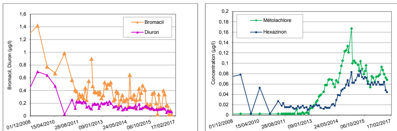
Illustration 29 : Fluctuations mensuelles mesurées sur Basse Pointe – Rivière Falaise pour différents pesticides (les valeurs inférieures à la limite de quantification sont représentées comme égales à LQ/2)
