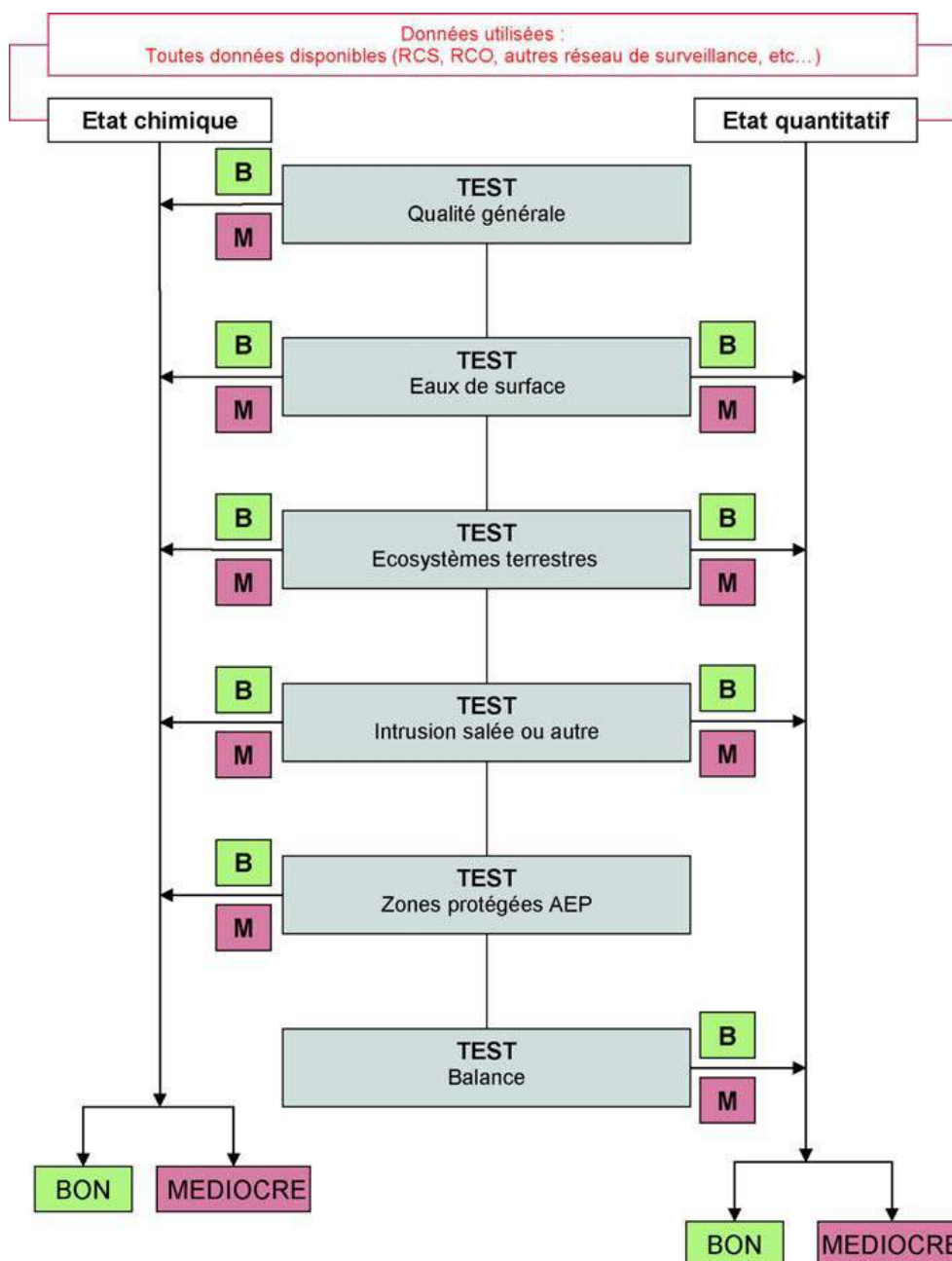
Illustration 4 : Tests de classification pour l'évaluation de l'état quantitatif et qualitatif
